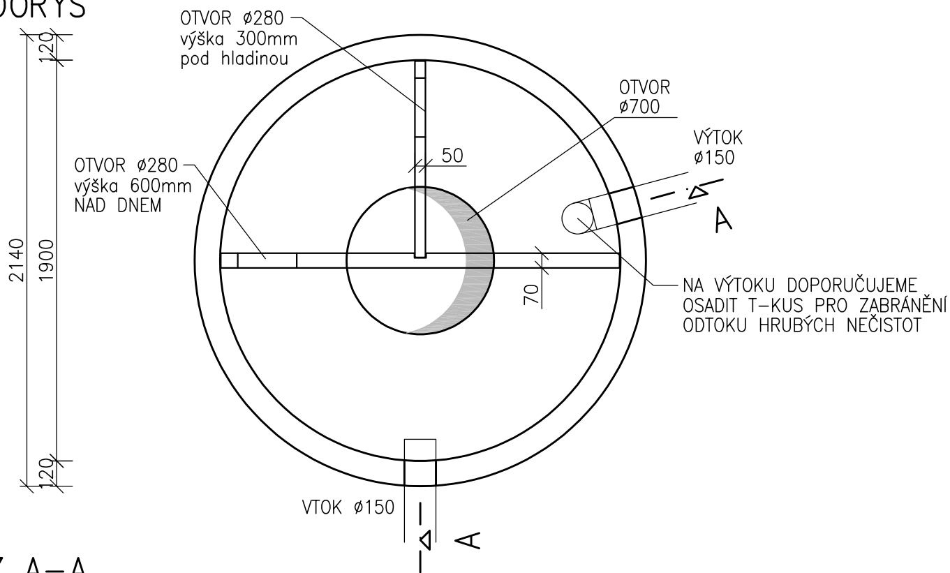
PŮDORYS
