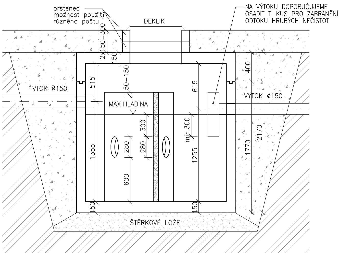
ŘEZ A-A
