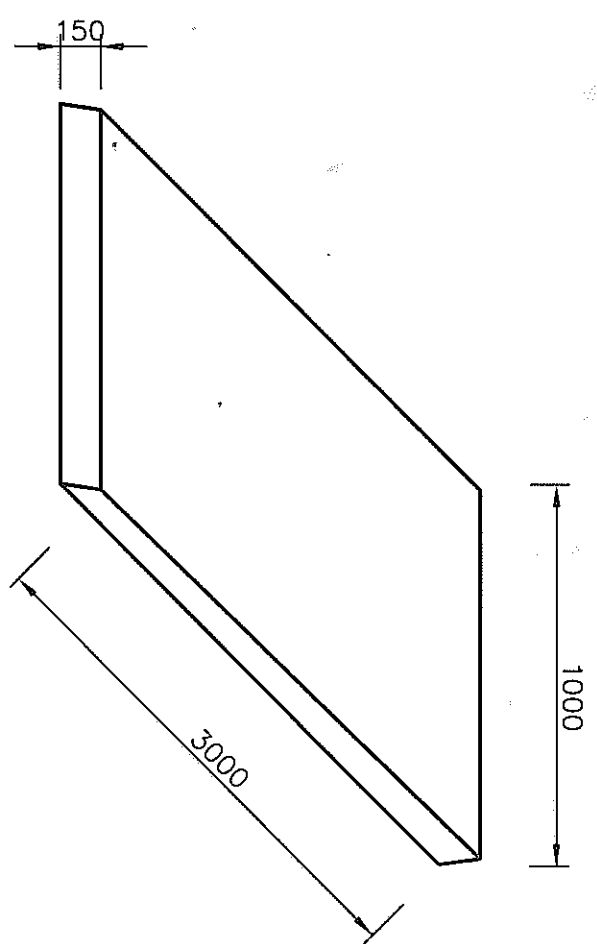
SILNIČNI PANEL KZD 300/100/15
